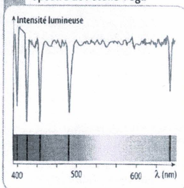
D Spectre de l'étoile Véga
